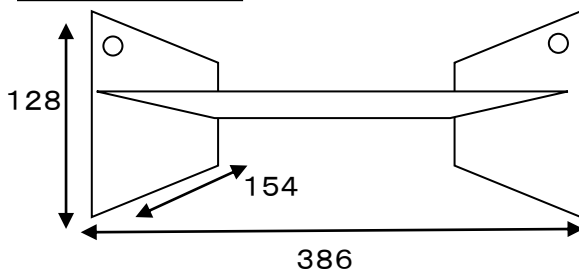
スタンド寸法
