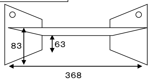
スタンド内側寸法
